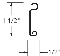
F-158 Slat
